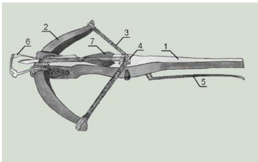
Obr. 1 Kuše – 1 socha, 2 lučičtě, 3 tětiva, 4 ořech, 5 spouštěcí páka, 6 třmen pro přišlápnutí kuše k zemi, 7 šípka
