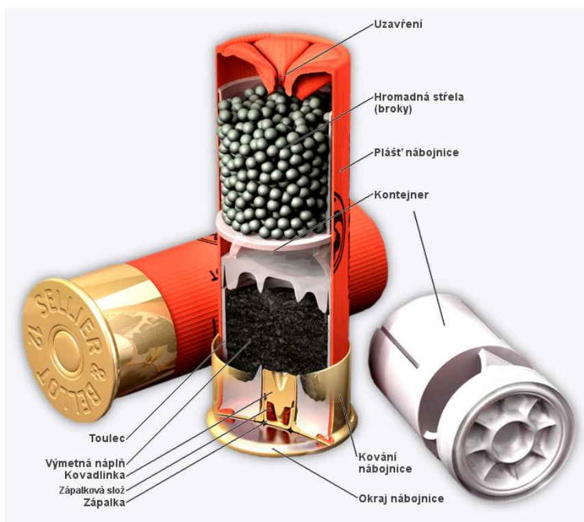
Obr. 6. Průřez brokovým nábojem s hromadnou střelou a středovým zápalom https://zbranekvalitne.cz/zbrojni-prukaz/nauka-o-strelivu
