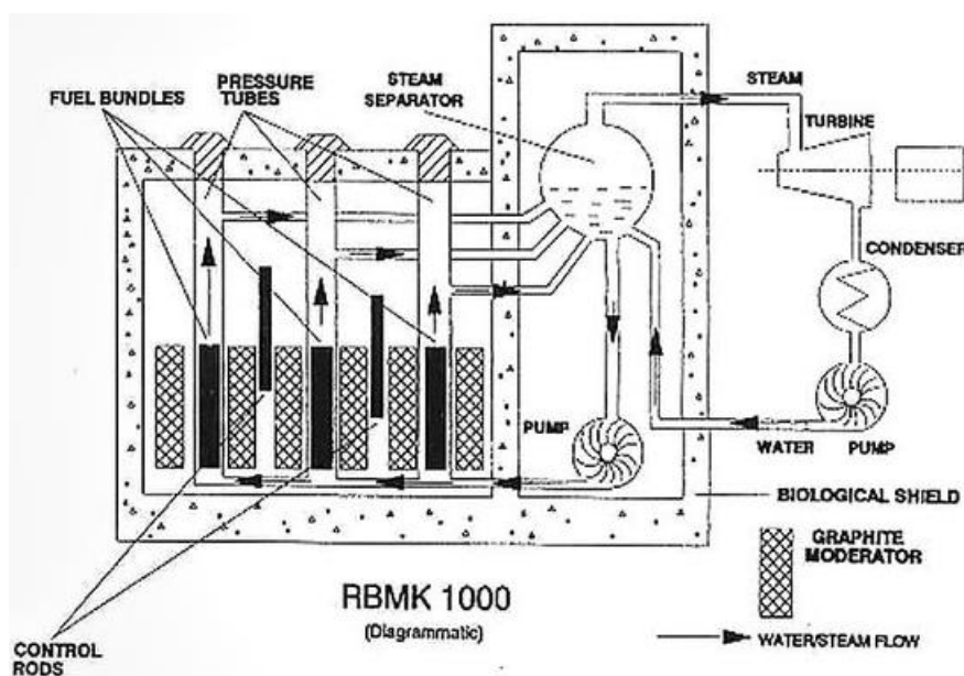
Obr. 1: Znázornění výrobního bloku Jaderné elektrárny Černobyl 10
