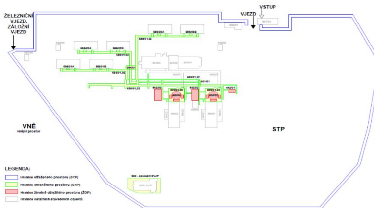
Obr. 2: Členění prostor Jaderné elektrárny Temelín z hlediska fyzické ochrany 25
