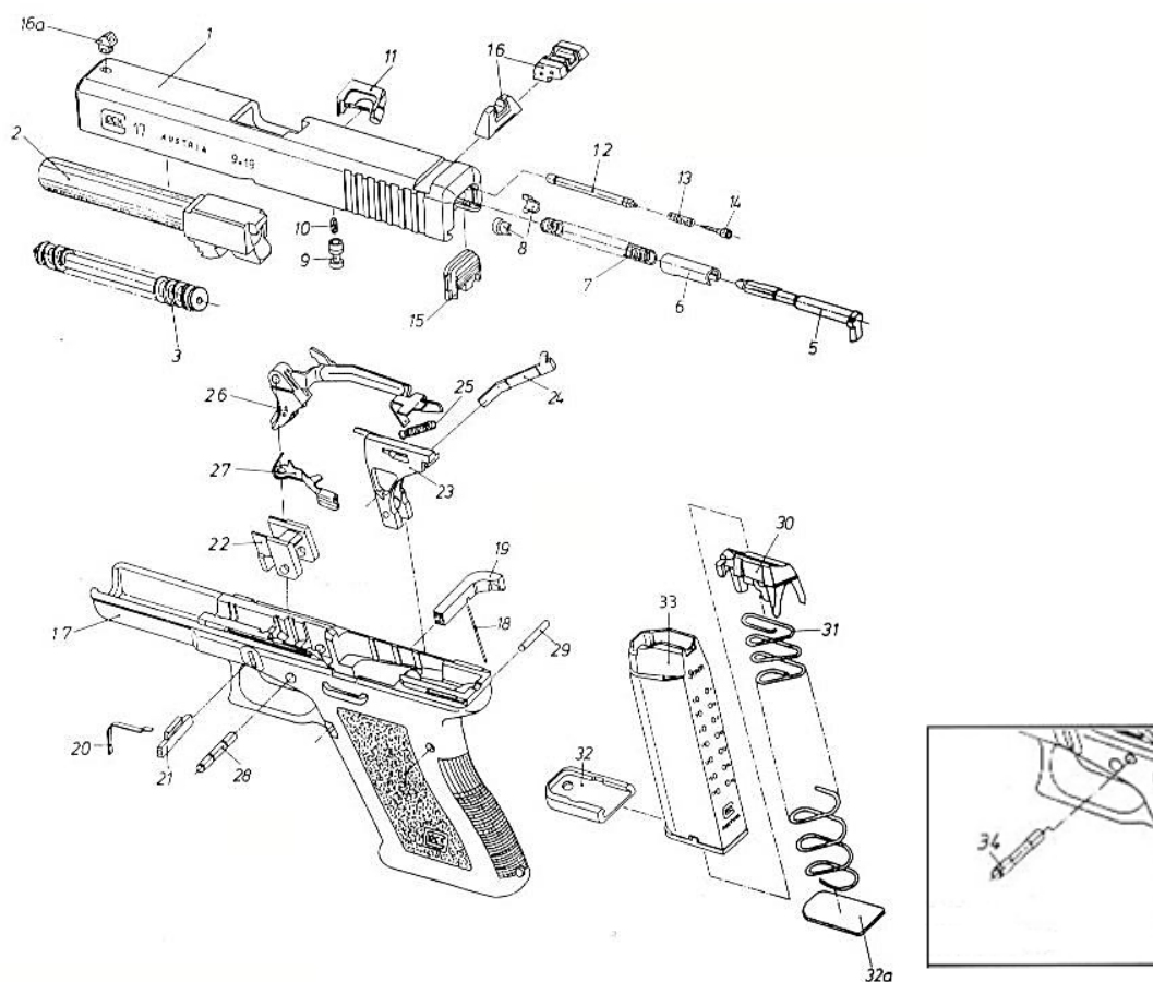
Obrázek 33 Technický nákres pistole Glock 17 168
