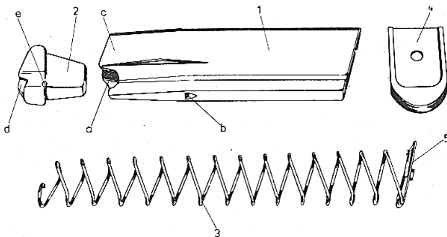
Obrázek 31 Technický náčrt rozloženého zásobníku pistole CZ 82 165
