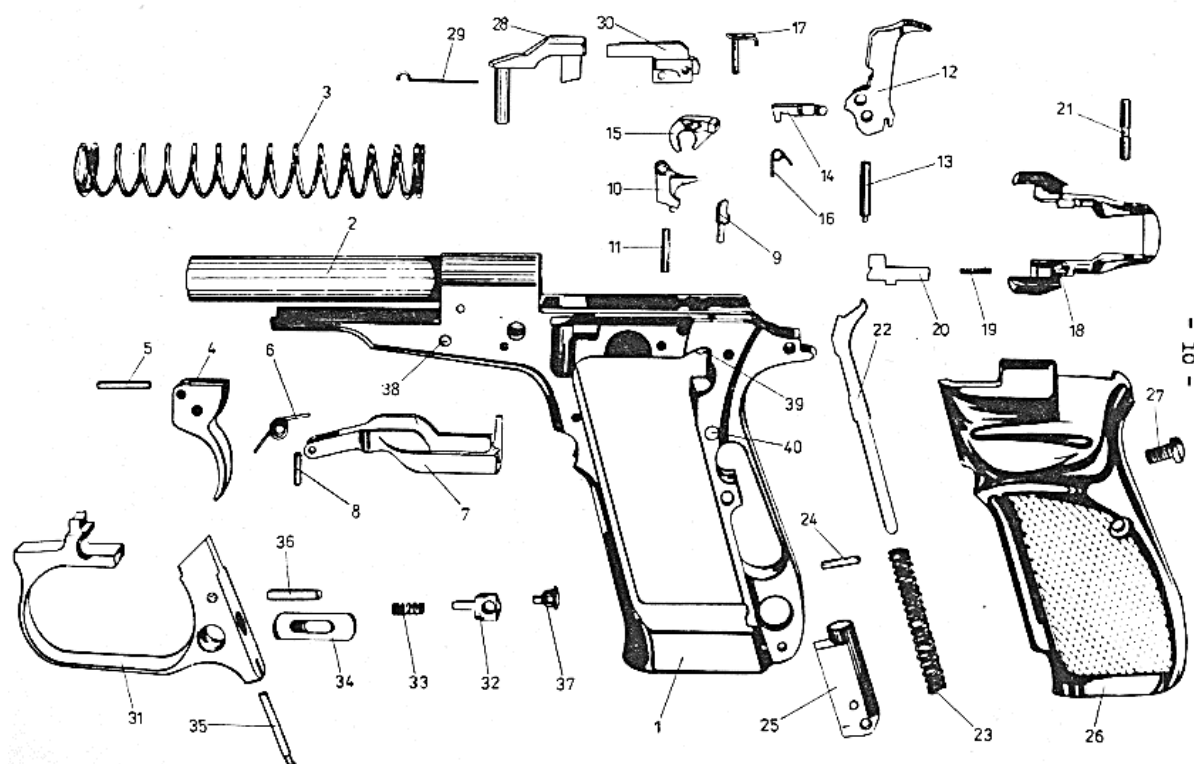
Obrázek 29 Technický náčrt pistole CZ 82 bez závěru 161
