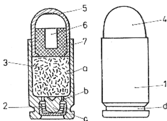
Obrázek 46 Technický nákres pistolového náboje 9 mm 181
