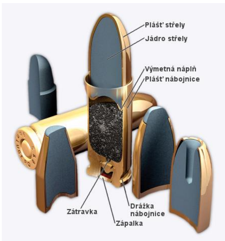
Obr. 3: Řez nábojem se středovým zápalem 67
